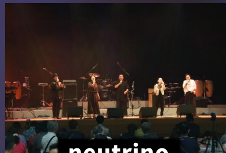
neutrino
